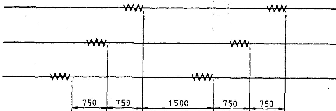
H.V. HORIZONTAL CONSTRUCTION
